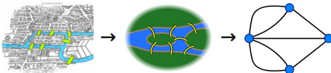
Könisberg-eko zazpi zubiak eta Eulerren teorema ( Wikipedia )
